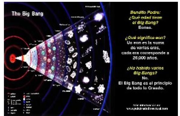
La edad del Big Bang
