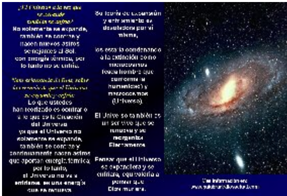
Se expande y se contrae
