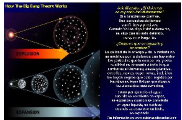
El Universo se expande y se contrae
